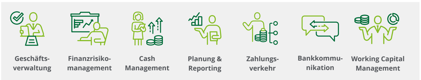
Abb. 1 – Business Prozesse
